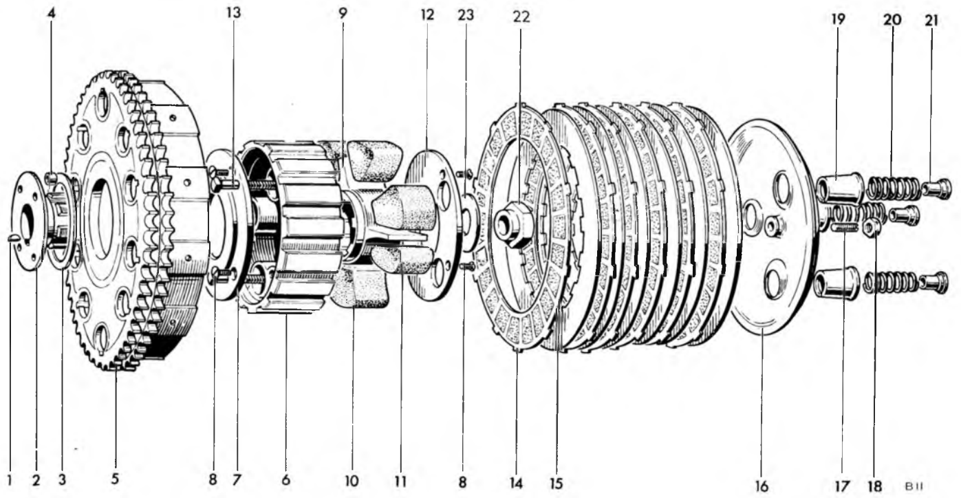
Fig. 12. CLUTCH
