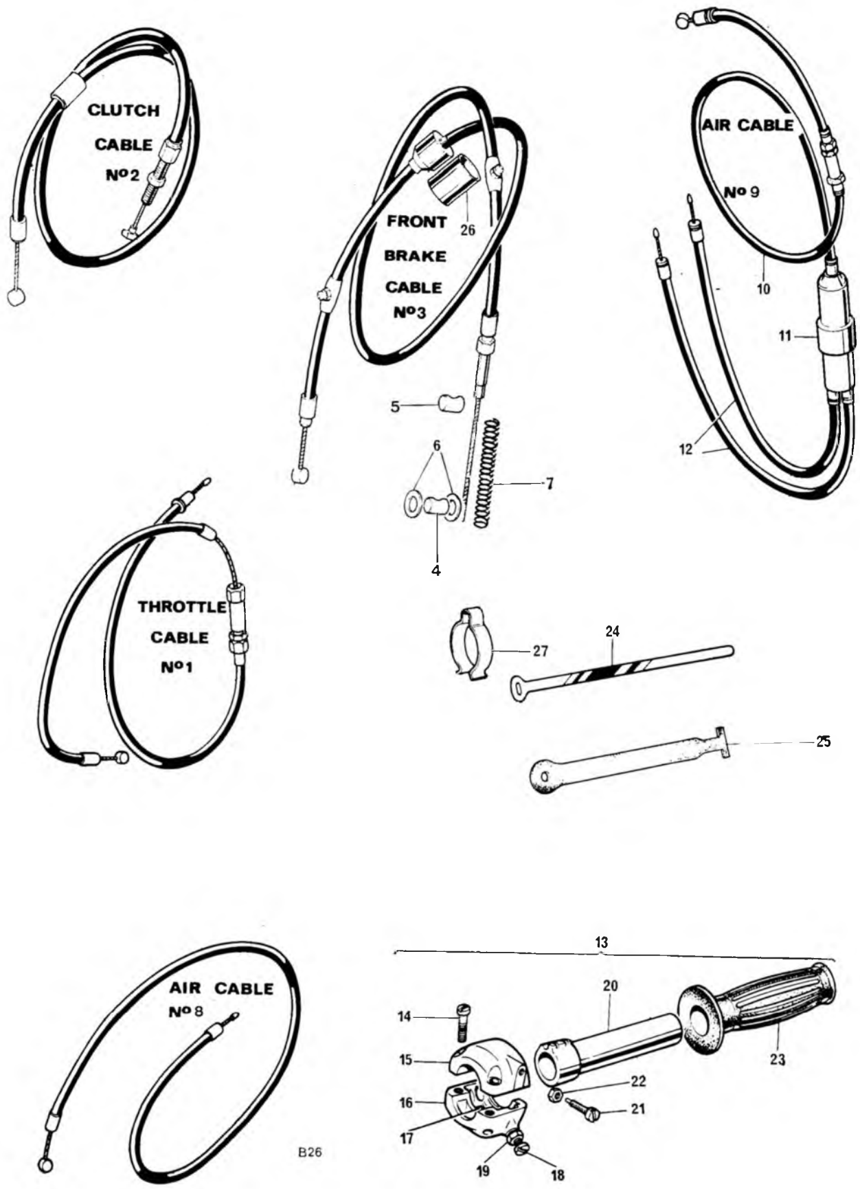
Fig. 27. CONTROL CABLES
