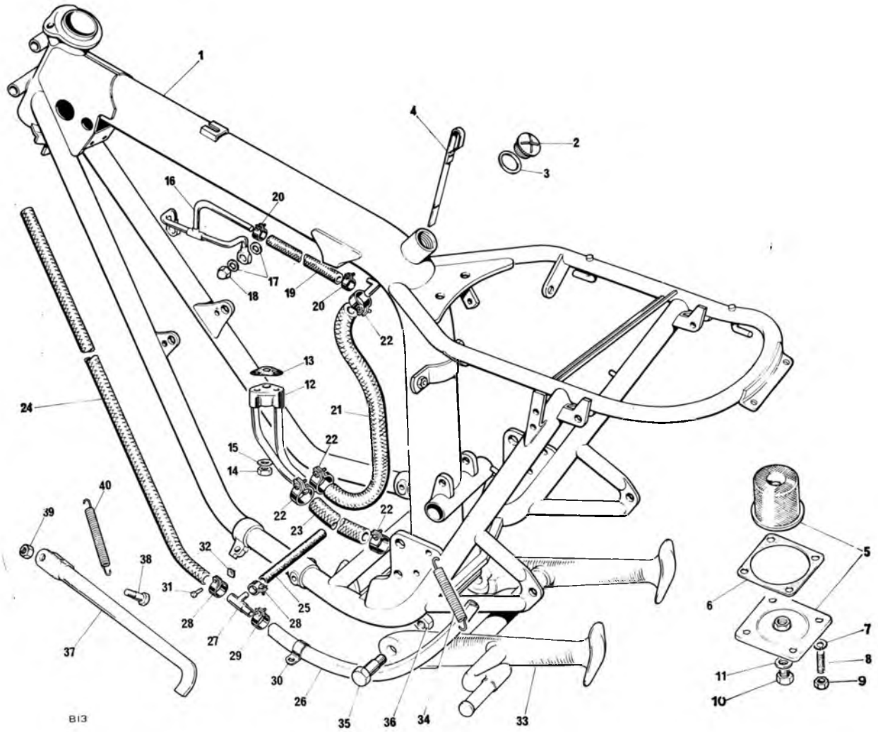
Fig. 14. FRAME
